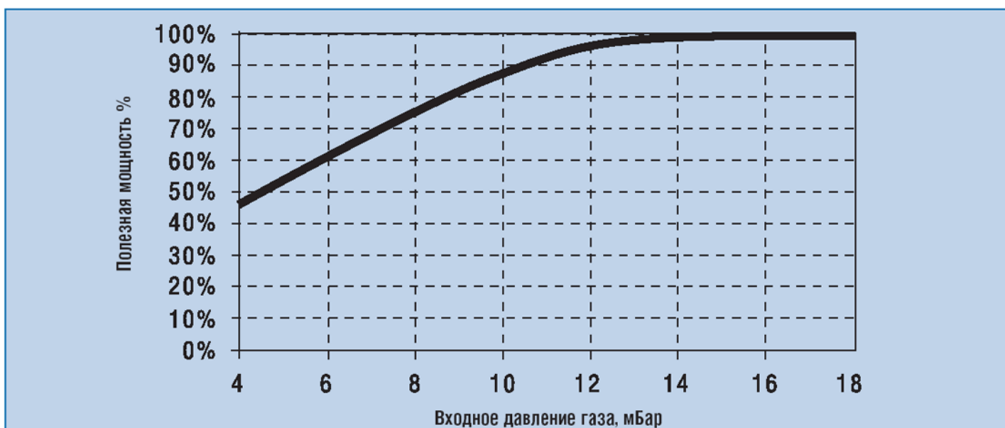
ГРАФИК ЗАВИСИМОСТИ ПОЛЕЗНОЙ МОЩНОСТИ ОТ ВХОДНОГО ДАВЛЕНИЯ ДЛЯ КОТЛА MAIN 24 FI.
