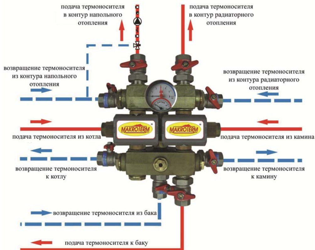
Рис.2: СХЕМА ПОДКЛЮЧЕНИЯ К ИНТЕГРАТОРУ I
