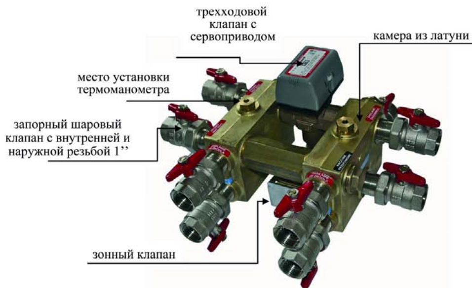
Рис.3: ОПИСАНИЕ ИНТЕГРАТОРА II
