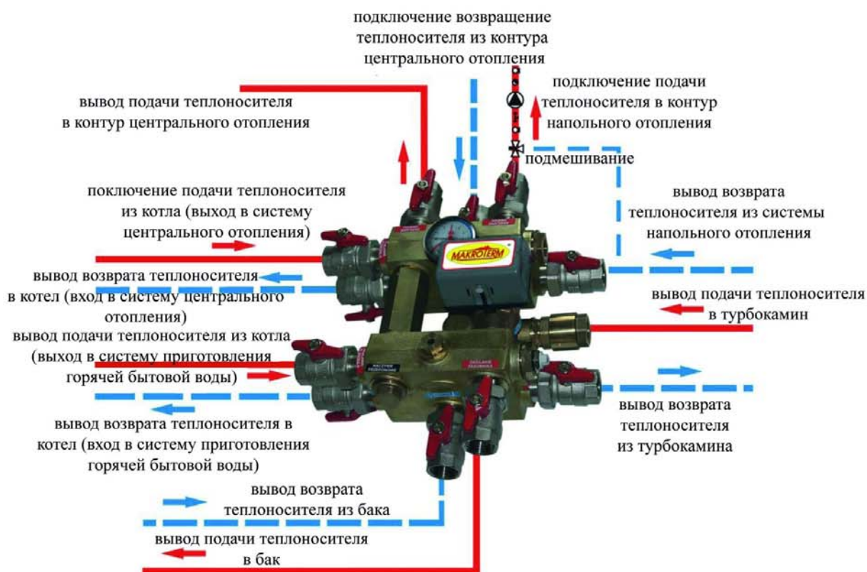
Рис.4: СХЕМА ПОДКЛЮЧЕНИЯ К ИНТЕГРАТОРУ III
